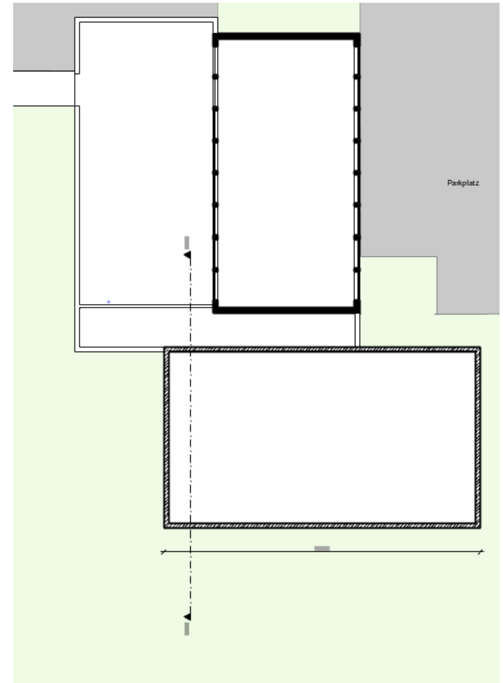
Obergeschoss
