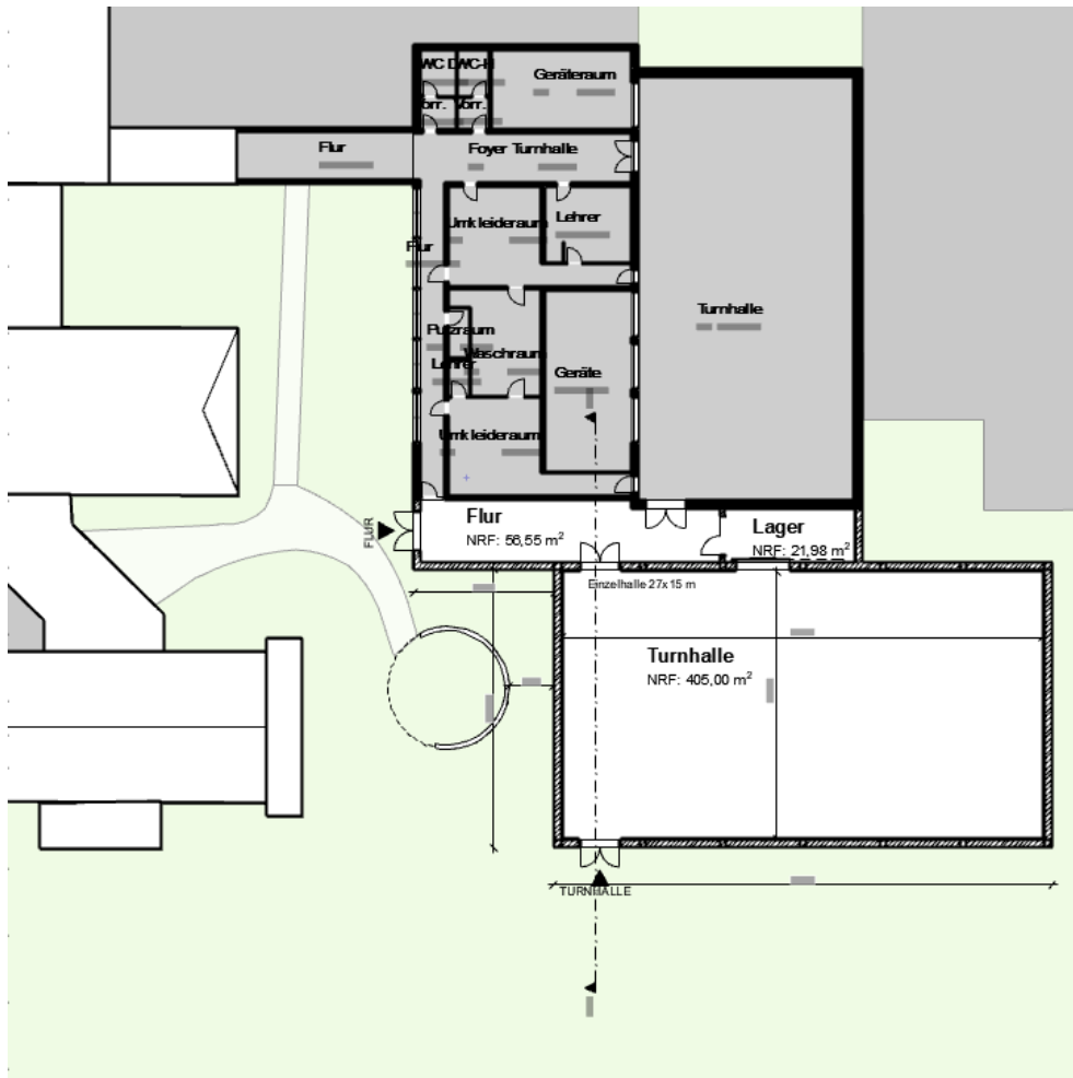
Erdgeschoss
